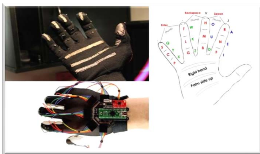
Εικόνα 11. Οι δύο όψεις του Keyglove και τα σημεία πίεσης που αντιστοιχούν στο πληκτρολόγιο
